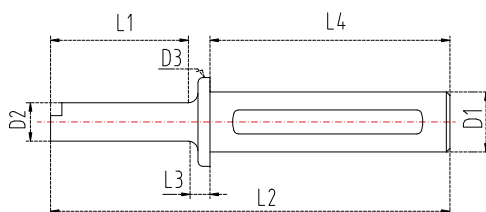
FIG. 2 PORTA INSERTO (UT) ДЕРЖАВКА (UT)
