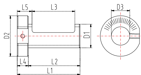
FIG. 3 - BUSSOLA ECCENTRICA (B) ВТУЛКА (B)
